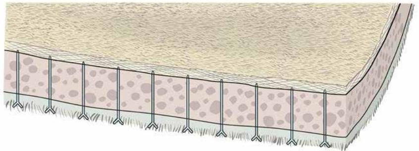
Skiss Bentonitmatta
