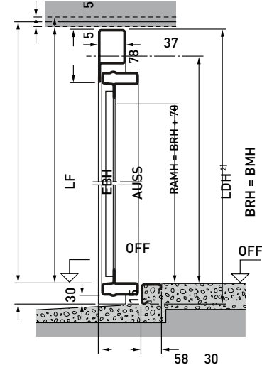
Vertikalsnitt Port med nedre anslag
