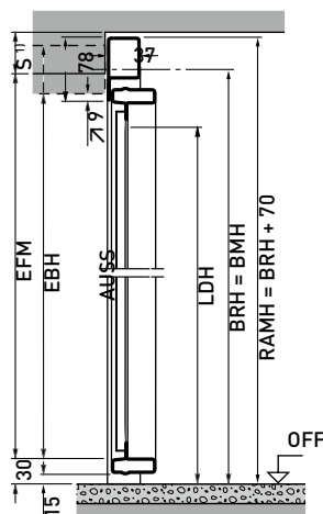
Vertikalsnitt Port med nedre anslag
