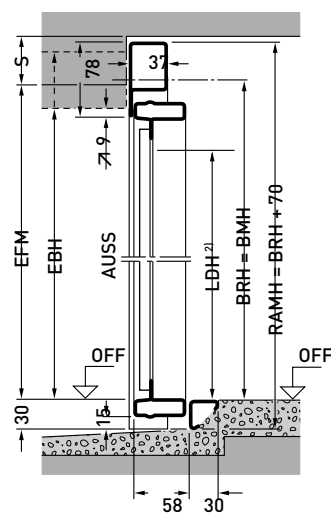
Vertikalsnitt Port med nedre anslag
