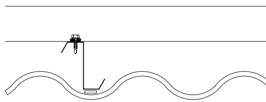
Figur 5.16 Infästning av Plannja Kombiläkt till ströläkt för eternitrenovering
