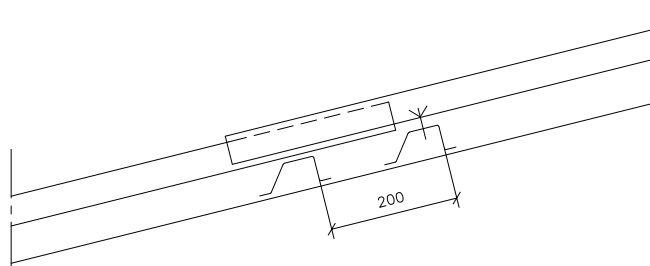
Figur 4.5 Dilatationsskarv
