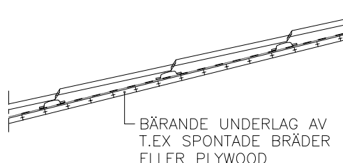
Figur 3.1 Plannja Renoveringsläkt på panel
