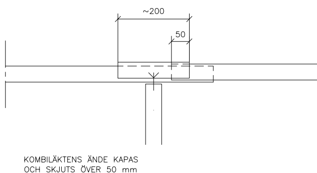
Figur 4.6 Dilatationsskarv Plannja Kombiläkt
