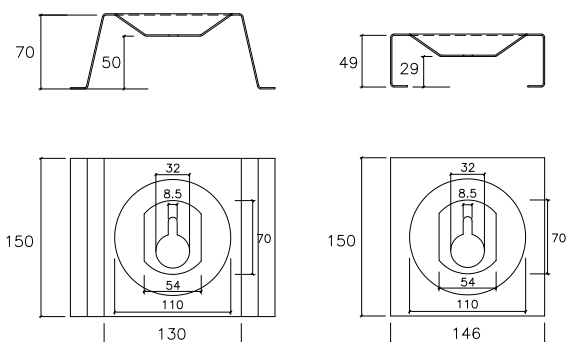
Figur 5.10 Plannja stödbricka för P6 resp. P8
