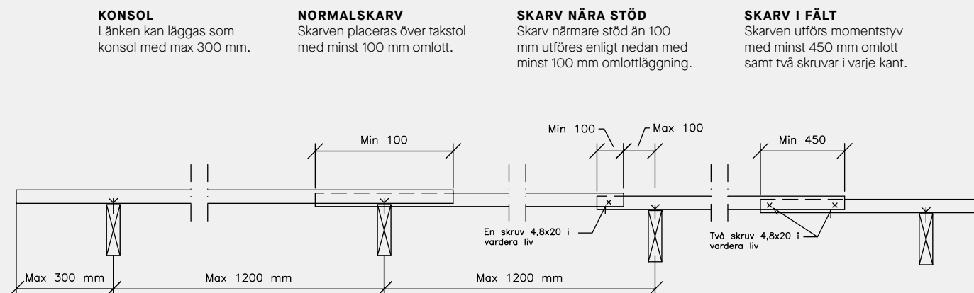
Figur 4.2 Skarvning av kombiläkt
