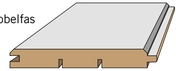
Råplan klyvsida
