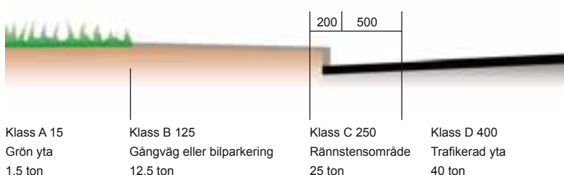
Hållfasthetsklassning av betäckningar enligt SS-EN 124
