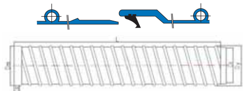
Rörkonstruktion Ø 1200—2500 PE
