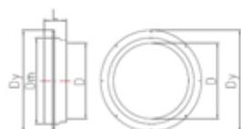
Ingjutningsmuffar Ø 600 – Ø 2500
