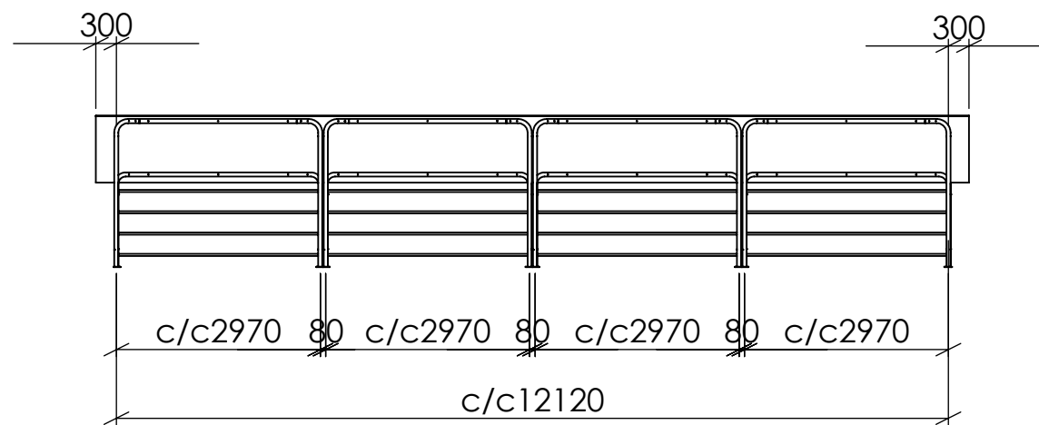
FRONTVY
