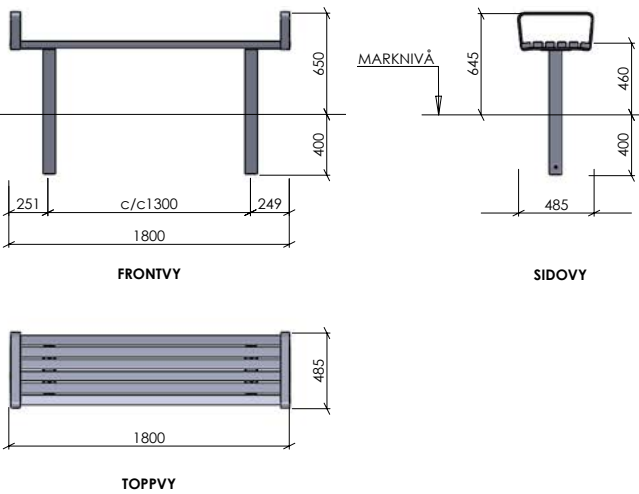
BÄNK
