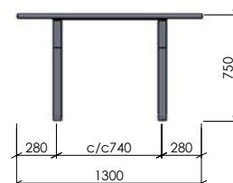
FRONTVY
