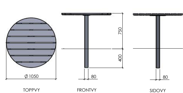
RUNT BORD
