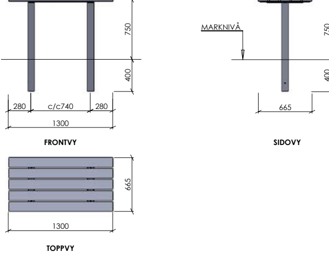
BORD
