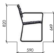
SIDOVY
