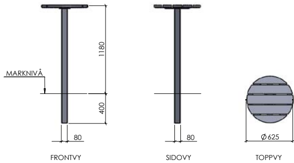
RUNT STÅBORD
