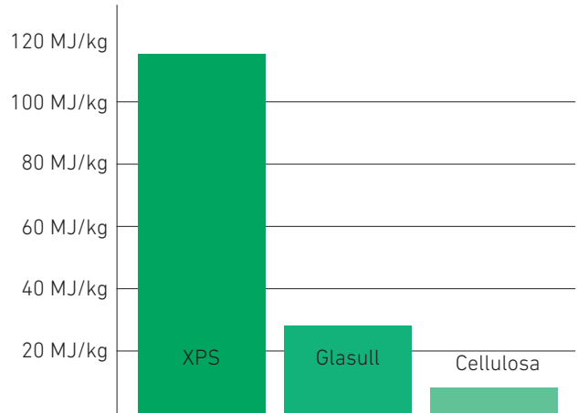
Primär energiförbrukning i produktionen av isoleringsmaterial i jämförelse. Källa: TU Graz
