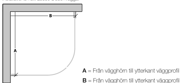
Installationsmått Lusso Duschväggar
