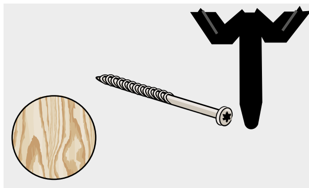
webertherm 406 skruv + webertherm 315 fäste
