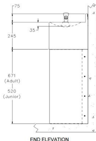
END ELEVATION
