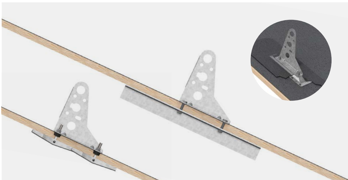
Motlägg, snabbfäste och fästplatta.
