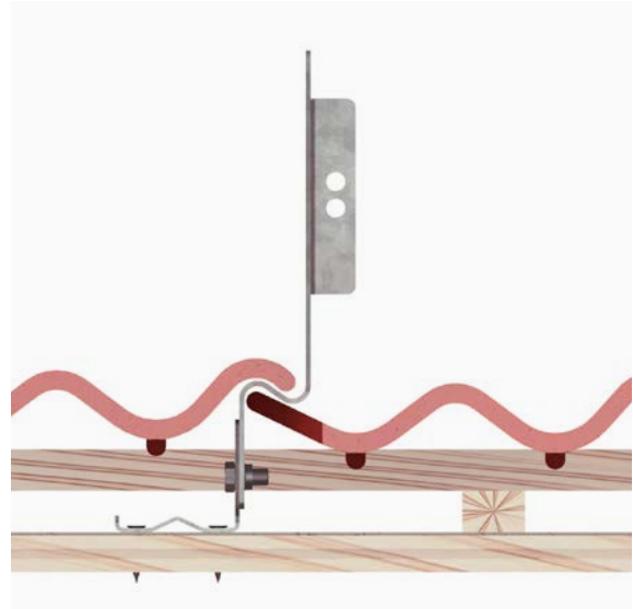
Hållare för svenskt lertegel sedd i tvärsektion.
