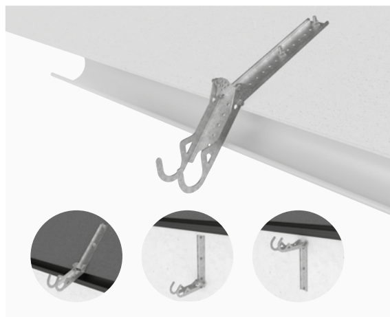
Glidskydd krok dubbel monteras på sarg/takkant utan ränna eller till takstege.
