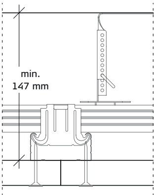
C-profilsystem, upphängt med Nonius-fäste.
