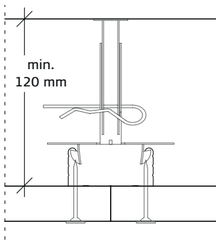
C-profiler, upphängda med Nonius-fäste.
