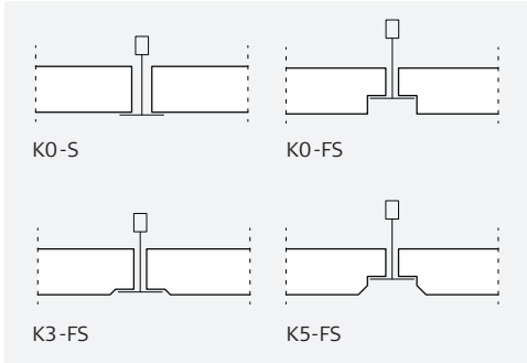
Montering med synliga T-profiler
