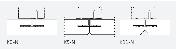
Montering med dolda KN-beslag på C60-profiler
