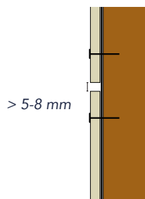
Underkonstruktion av trä, öppen vågrät fog
