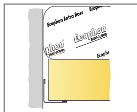
Absorber villar på vägglister
