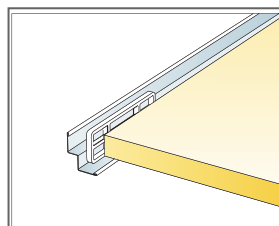
Connect väggdistanst 5 för fixering av passbitar
