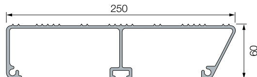
Stegprofil 250/60 , max längd: 2350 mm
