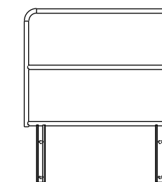
Räcke för bryggsektion 1,5 m 100911/8024327 inkl. 4 st kopplingsbeslag 201040SS
