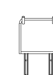
Räcke för bryggsektion 1 m med spöhallare 100920/8024332 inkl. 4 st kopplingsbeslag 201040SS
