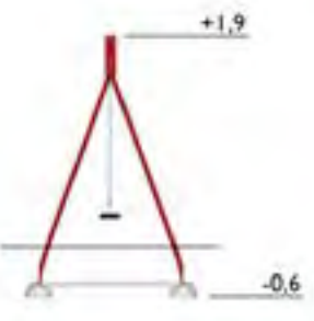
Gungställning i stål Nedgrävningsfundament
