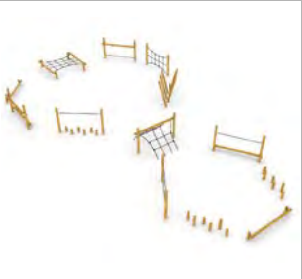
Hinderbana L 8061281 naturell ✚ 20,0 x 12,3
