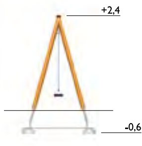
Gungställning i trä Nedgrävningsfundament
