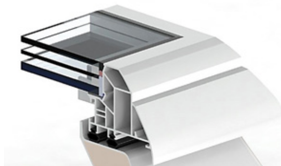
Plan profil – inga vattenansamlingar, inga smutsfällor.
