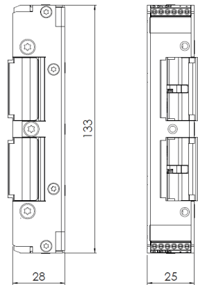
Måttskiss STEP 92 Preload.
