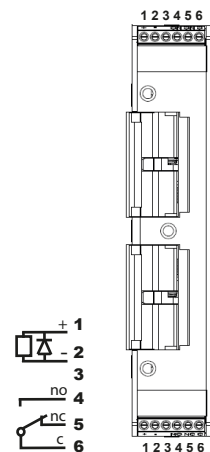
Kopplingsschema med kolvkontakt. Inkoppling sker med skruvplintar.
