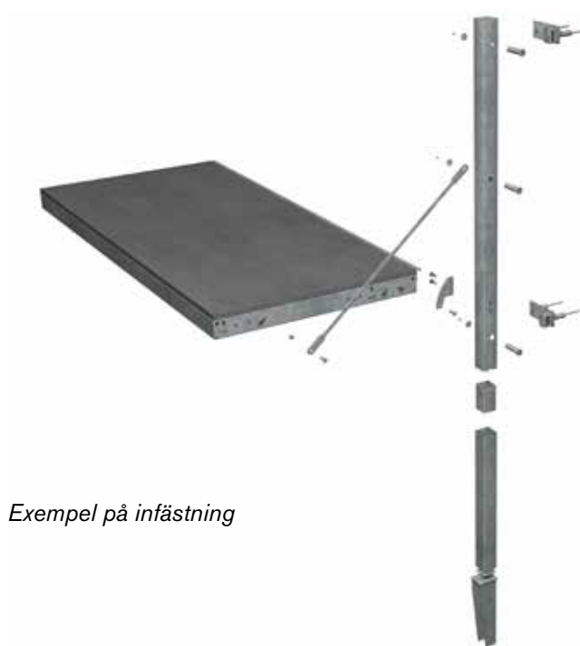
Infästning med dragstag
