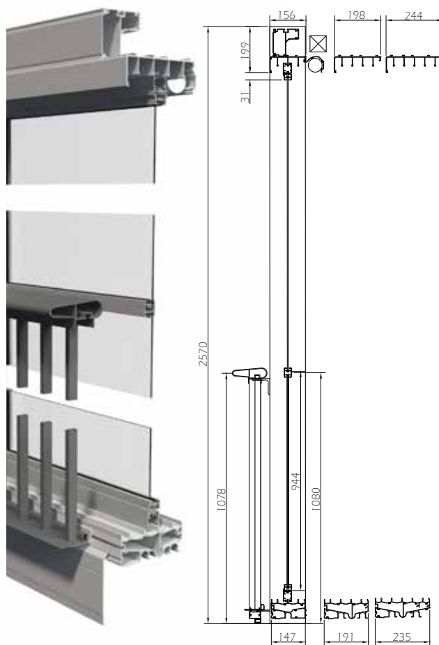
Space. Tvärsnitt och ritning från sidan.
