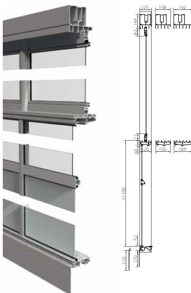
Access. Tvärsnitt och ritning från sidan.
