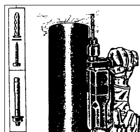
Bild 7. Dra tillbaks brandmanschetten och borra hålen. Tryck manschetten tillbaka mot väggen/bjälklaget och fäst med rekommenderade plugg, skruv eller ankare.
