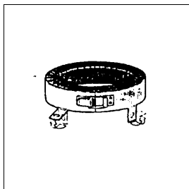
Bild 2. Bøj fäsklämmorna 90° ut med hjälp av en plattång.
