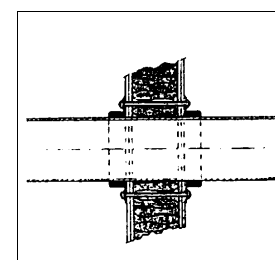
Bild 8. KBS PIPESEAL C kan också installeras i lättväggar (se bilaga C04). Vi denna typ av installation fästes manschetten med M6 till M8 genomgående trådbult med bricka (alternativt gipsexpander).
