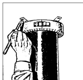
Bild 6. Tryck brandmanschetten mot väggen eller bjälklaget och markera borrhålen i fästbyglarna.
