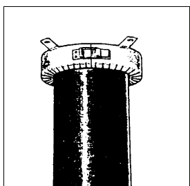
Bild 5. Stäng bygellåset när manschetten monterats på röret (se till fjädermekanismen låses).
