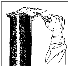
Bild 1. Gapet mellan plaströr och vägg/bjälklag skall fyllas med t.ex obrännbart bruk, stenull eller KBS FOAMCOAT C11. Om stenull används bör spalten vara max 15 mm bred.
