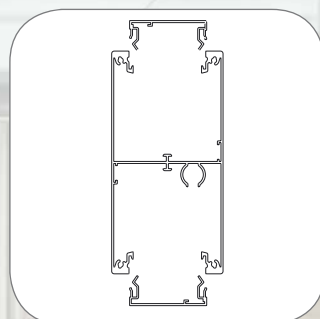
Dubbelsidig profil 65x130 mm, front 45 mm
