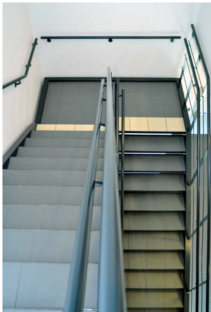
Logistikcentral i Torslanda. Rak trappa i tre löp. Trappstegen och planerna är belagda med klinkers. Första steget i varje löp har kontrastmarkering. Floby Durk har utfört montaget.
