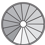
15 steg/varv Radi 700 - 1000
