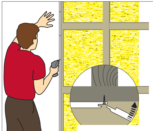
Skivan skruvas eller spikas dolt. Lim behövs inte.
