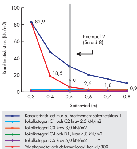
Karakteristisk ylast krav och kapacitet för Compactfloor lokalkategori C och D1
