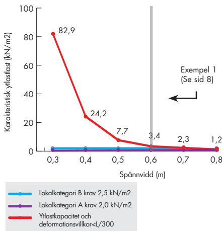
Karakteristisk ylast krav och kapacitet, Compactfloor P6, lokalkategori A, B
