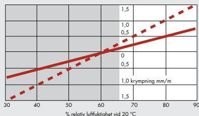
Aktuellt fuktområde för skivor i klimatklass 1
