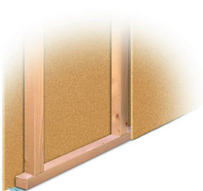
EI 15. Väggar med stomme av träreglar min. 45x45 mm c ≤600 mm, på båda sidor försedd med Byggelits 12 mm spånskivor.
