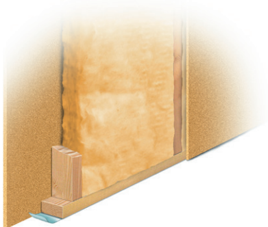
EI 30. Vegg med stomme av träregrar min. 45x70 mm c ≤ 600 mm, på båda sidor försedd med Byggelits 12 mm spånskivor. Mellan reglarna ska finnas min. 70 mm isolering av stenull.
