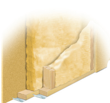
EI 60. Vegg med dubbel träregrarstomme eller korsande reglar min. 45x70 mm c ≤ 600, på båda sidor försedd med Byggelits 12 mm spånskivor. Mellan reglarna ska finnas min. 2x70 mm isolering av stenull.
