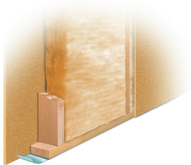
EI 30. Vegg med stomme av träregrar min. 45x95 mm c ≤ 600 mm, på båda sidor försedd med Byggelits 12 mm spånskivor. Mellan reglarna ska finnas min. 95 mm isolering av mineralull.
