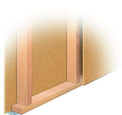
EI 30. Väggar med stomme av träreglar min. 45x70 mm c ≤600 mm, på båda sidor försedd med Byggelits 12 mm spånskivor.
