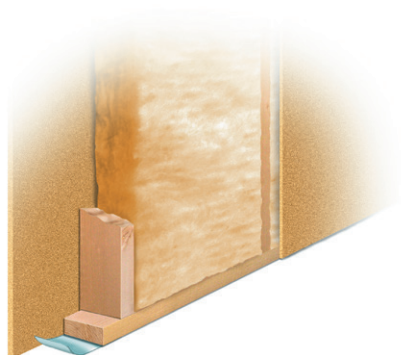
R 30. Väggar med stomme av träreglar min. 45x95 mm, c ≤600 mm, på båda sidor försedd med min. Byggelits 18 mm*) spånskivor. Träreglarna ska vara avstyvade med kortlingar eller likvärdigt åtminstone på mitten. Mellan reglarna ska finnas min. 95 mm isolering av mineralull.
