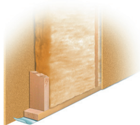
REI 30. Väggar med stomme av träreglar min. 45x95 mm c ≤600 mm, på båda sidor försedd med min. Byggelits 12 mm spånskivor. Mellan reglarna ska finnas min. 95 mm isolering av stenull.
