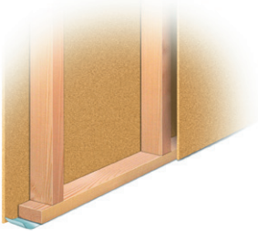
REI 15. Väggar med stomme av träreglar min. 45x70 mm c ≤600 mm, på båda sidor försedd med Byggelits 12 mm spånskivor.
