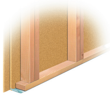
EI 30. Vegg med dubbla träregrar min. 45x70 mm c ≤ 600 mm, på en sida försedd med min. Byggelits 24 mm*) spånskivor.
