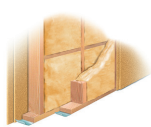
REI 60. Väggar med dubbel träregelstomme, min. 45x120 mm, c ≤600 mm, på båda sidor försedd med min. Byggelits 24 mm*) spånskivor. Träreglarna ska vara avstyvade med kortlingar eller likvärdigt åtminstone på mitten. Mellan reglarna ska finnas min. 2x120 mm isolering av mineralull.
