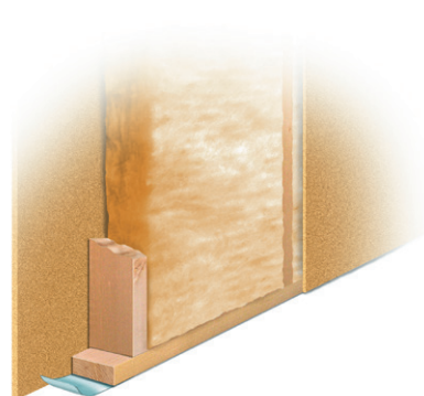
EI 60. Vegg med stomme av träregrar min. 45x95 mm c ≤ 600, på båda sidor försedd med Byggelits 12 mm spånskivor. Mellan reglarna ska finnas min. 95 mm isolering av stenull.
