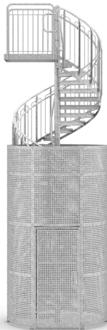
Skyddsbur i perforerad plåt
