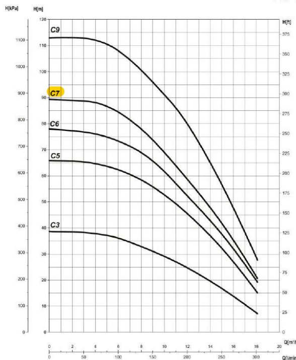
Kapacitetskurva pump SAER C/7 MBS 4,5 kW, 380-415V, 50Hz, 7,2A
