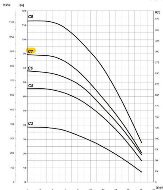
Kapacitetskurva pump SAER C/7 MBS 4,5 kW, 380-415V, 50Hz, 7,2A
