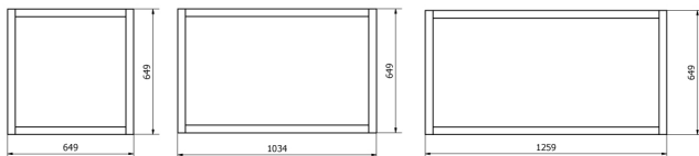
Höjd 649 mm
