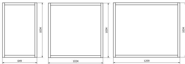
Höjd 1034 mm
