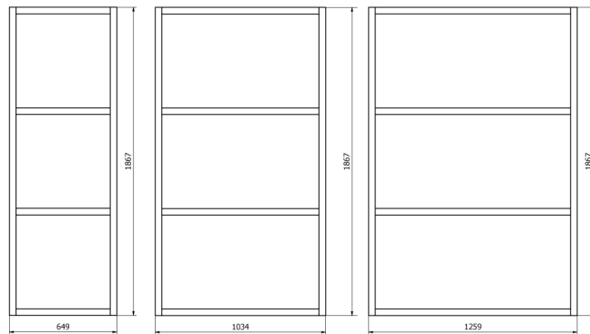
Höjd 1867 mm
