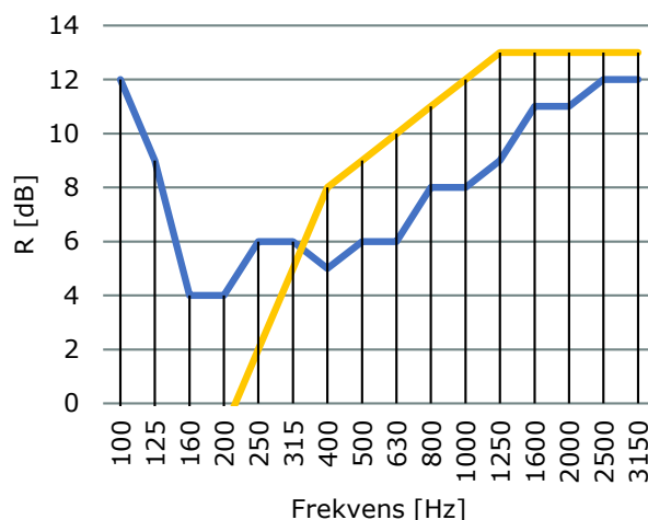
Reduktionstalskurva, medeldensitet
