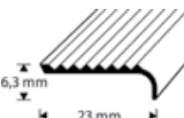
C10 Råfflad yta mässing
