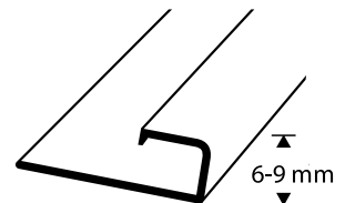
Kakelprofil H = 6 mm, 9 mm
