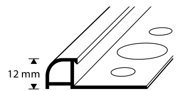
Kakelprofil H= 12 mm
