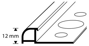
Kakelprofil H= 12 mm
