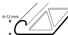
Kakelprofil H = 6 mm, 8 mm, 10 mm, 12 mm
