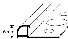
Kakelprofil H= 6 mm
