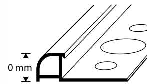
Kakelprofil H= 10 mm
