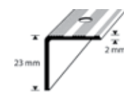
D5 Råfflad yta aluminium
