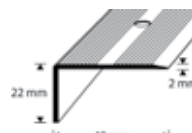
D7 Råfflad yta gold, silver, brons
