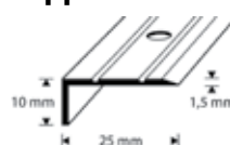
D1 Spårad yta guld, silver, brons
