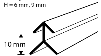
Kakelprofil pilmodell H = 10 mm
