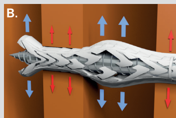
B. SXR-L vidgar sig i hålrum och skapar ett mekansikt stopp.
