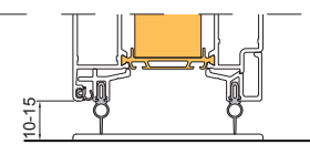
Dörr med släpplis i underkant. Godkänt vid rökastäthet S_a / S_m
