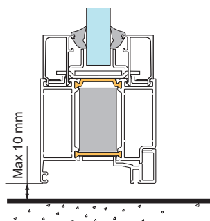
EI 30, EI 60 Utan tröskel 10 mm fritt till golv. EI 30 kompletteras med borstlist i underkant.
