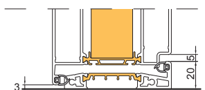
Dörr med med anslagstättning mot tröskel. Godkänt vid rökastäthet S_a / S_m
