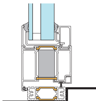
EI 30, EI 60 Tröskel 20 mm över golv med anslag.
