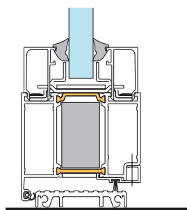
EI 30, EI 60 Tröskel 10 mm på golv med anslag.
