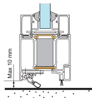
EI 30 Utan tröskel 10 mm fritt till golv med automatisk tätningströskel.
