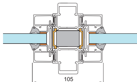
Vertikalspröjs vid partihöjd över 2300 mm
