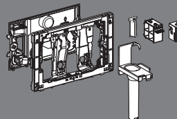
Geberit DuoFresh-modul med manuell aktivering och insats för Geberit DuoFresh doftstav
