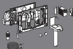
Geberit DuoFresh-modul med automatisk aktivering och insats för Geberit DuoFresh doftstav
