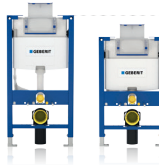
Geberit Omega inbyggnadscistern
